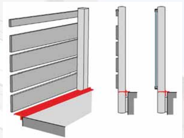
Trittspaltabdeckung bei Montage VOR Steher
