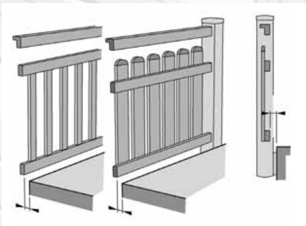
Trittspalt bei Seitenmontage (max 3-4 cm)
